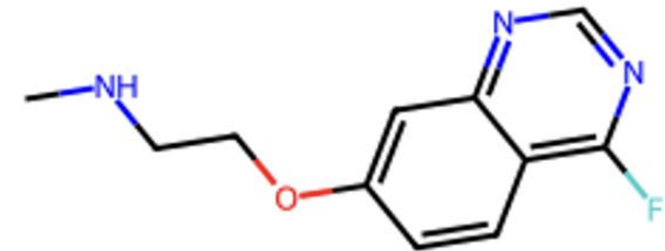
Молекул Б
